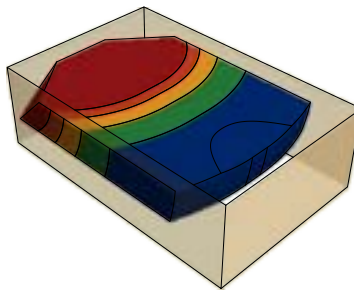
Tepelný účinok pri nahriatí 1 strany (6 x 4 m formát)
